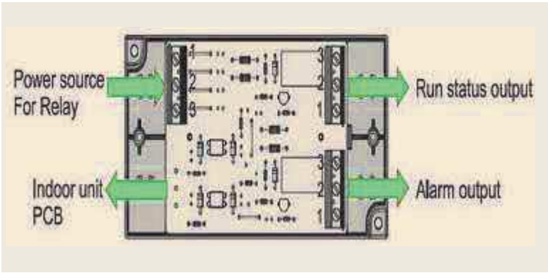
Reléový modul SPX-WDC8
