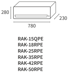
Vnitřní jednotky
