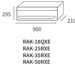
Vnitřní jednotky
